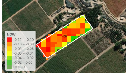
Imagen Humedad de Suelo Semana N° 28
